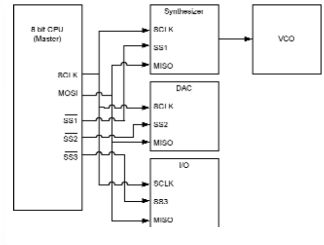
▶그림 11. SPI를 통해 제어되는 합성기
