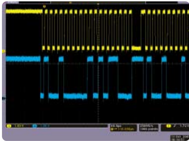
▶ 그림 3. I2C 버스에서 획득된 한 메시지
