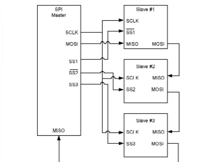
▶ 그림 9. 데이터 체인 방식의 SPI 구성
