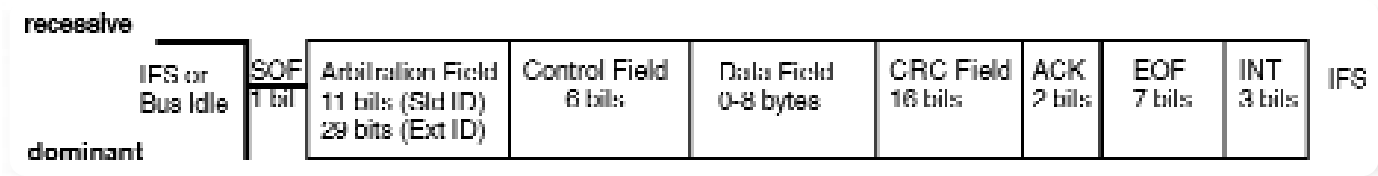
▶ 그림 14. CAN 데이터/원격 프레임
