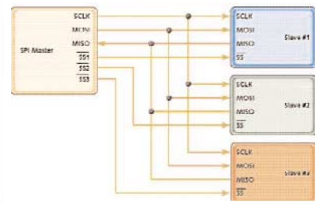
▶ 그림 8. 일반적인 SPI 구성
